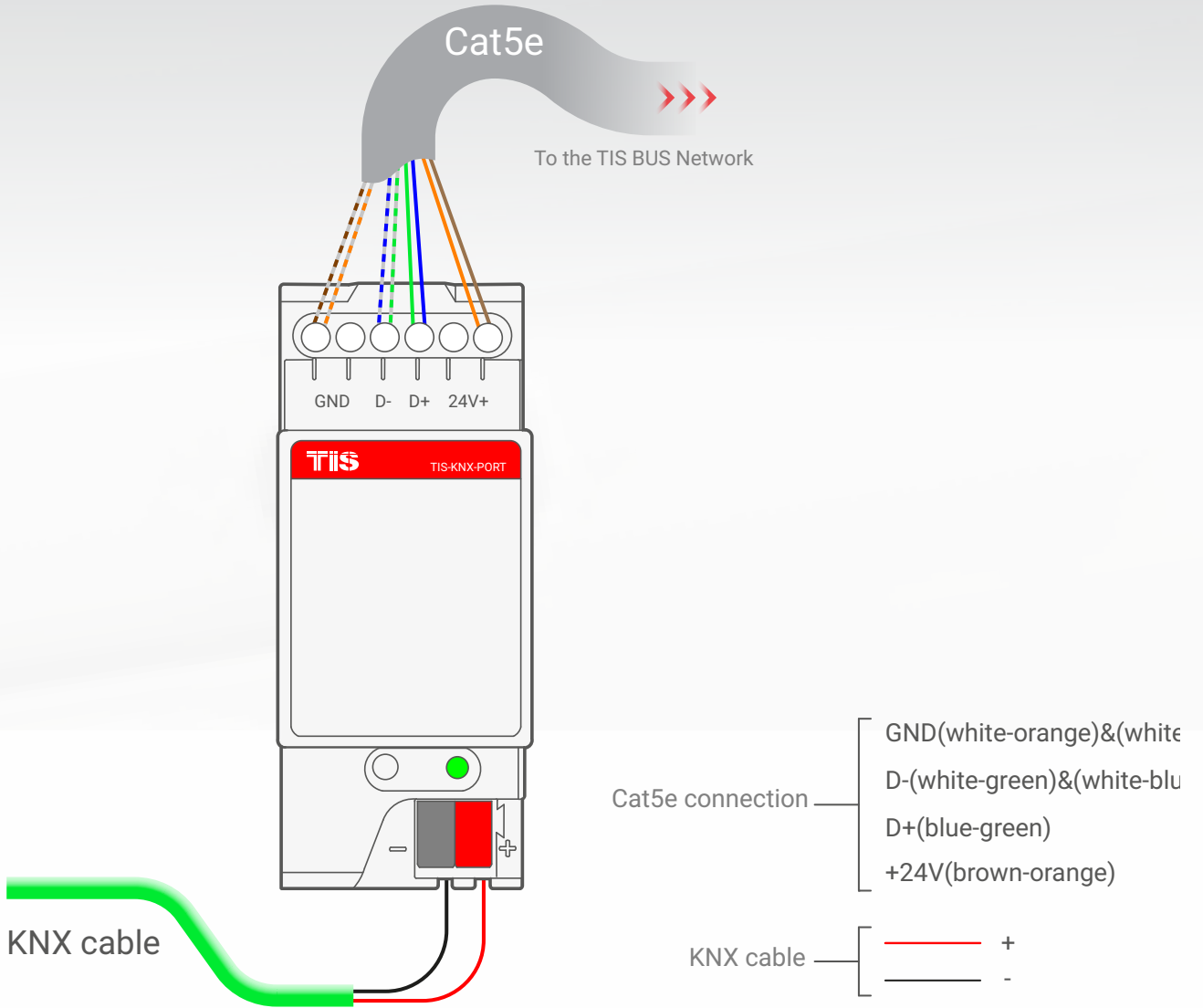
▲ TIS BUS-KNX Ağı Geçidi Bağlantı Diyagramı
