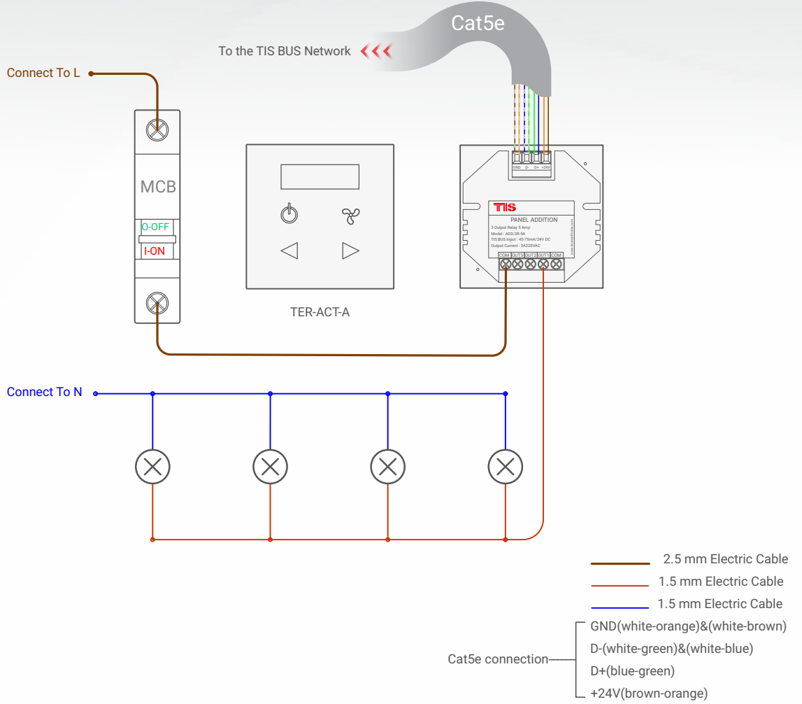
▲ TER-ACT-A ve ADD-3R-5A Aydınlatma Bağlantı Diyagramı
